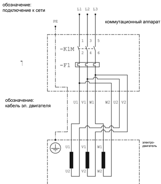
Рис. 6 / Схема 6: Соединение для прямого старта (DOL) для моторов со схемой звезда/треугольник – (соединение со всеми обмотками через сетевой кабель ) Соединение по схеме треугольник в обмотке
